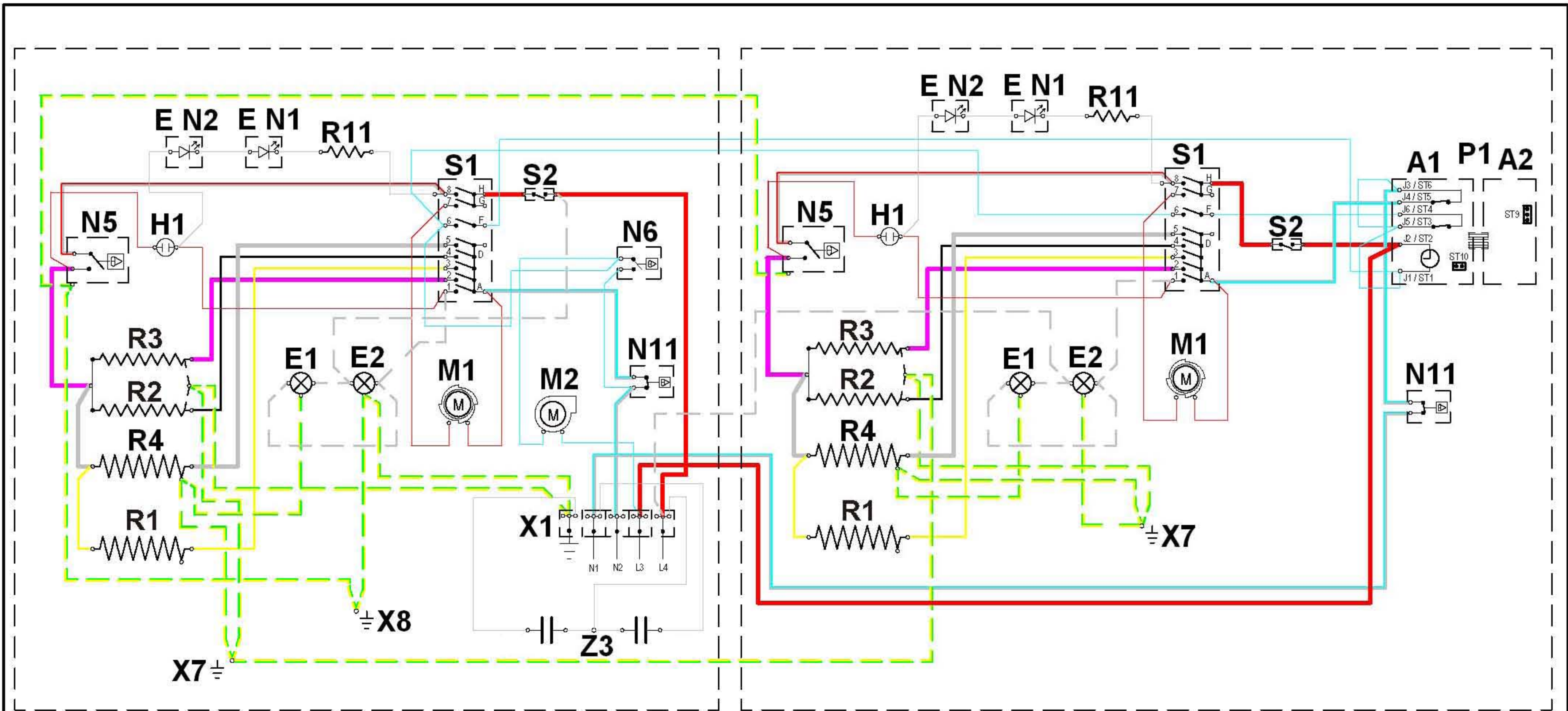
BACKOFEN OBEN
