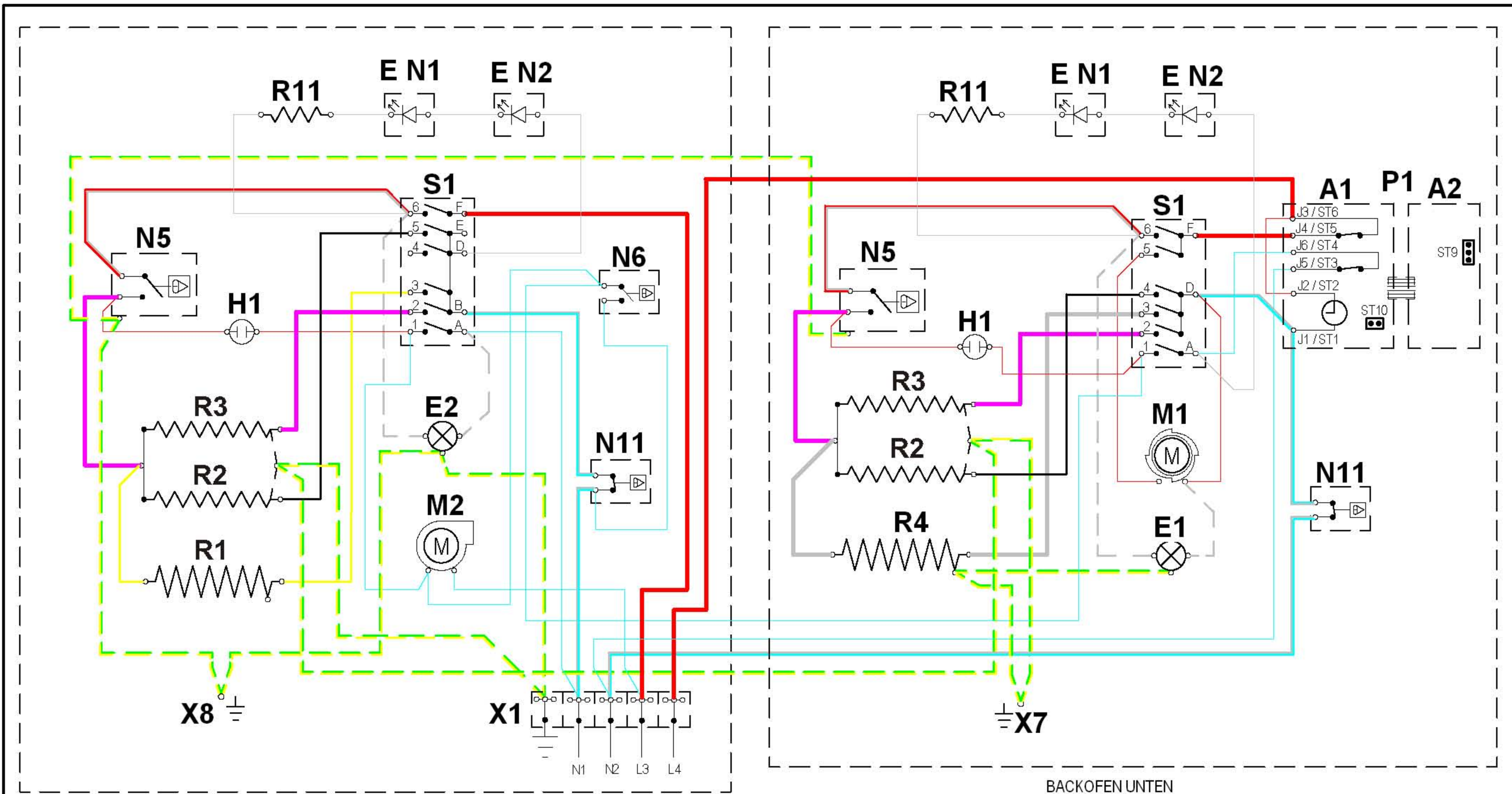
BACKOFEN OBEN
