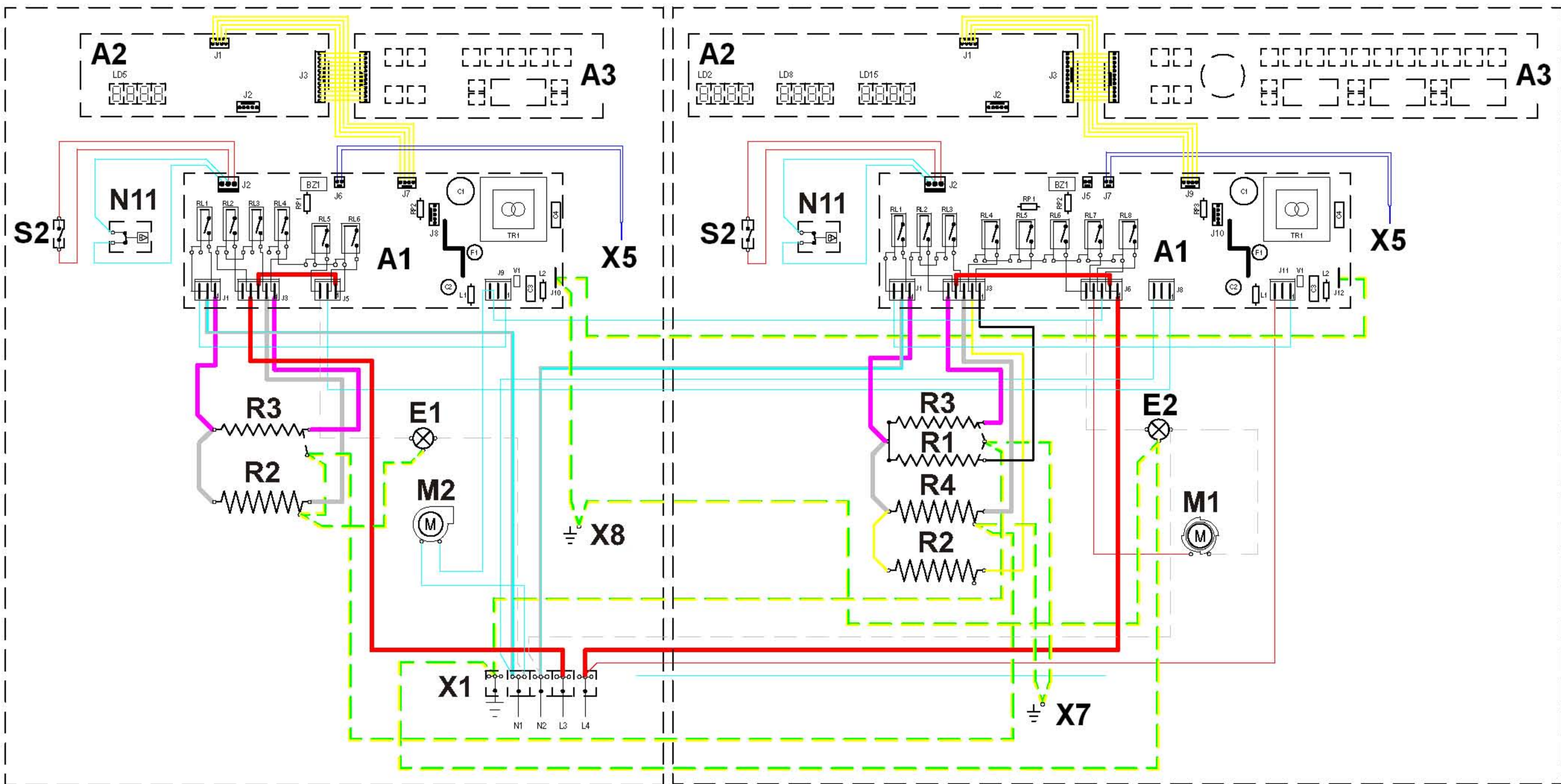
Backofen unten
