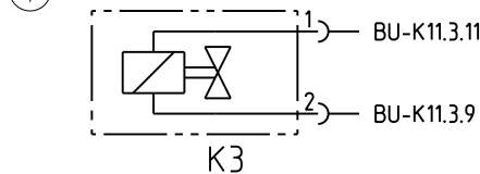
Auslassventil
