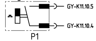
Flügelradzähler
