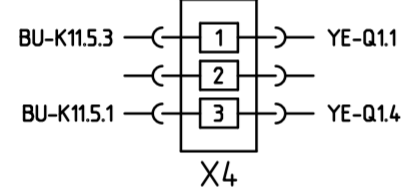
Kupplung
