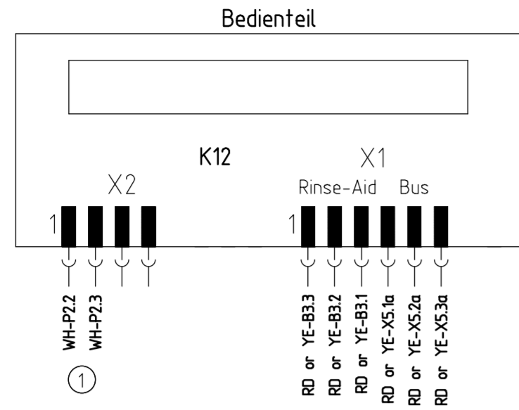
Sensor Klarspülmangel
