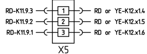
Kupplung
