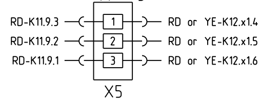
Kupplung
