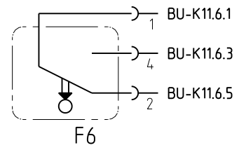
Schwimmerschalter
