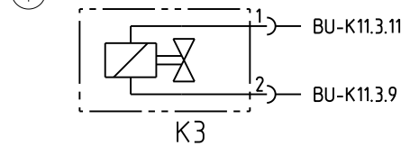
Auslassventil
