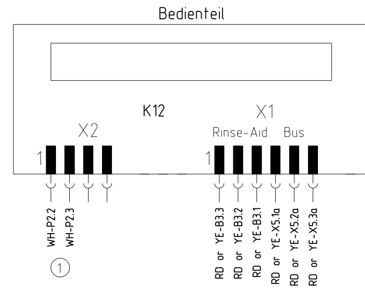
Sensor Klarspülmangel
