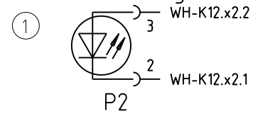
Betriebsanzeige
