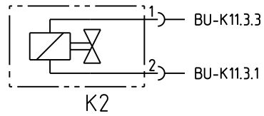
Füllventil
