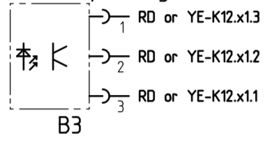
Sensor Klarspülmangel
