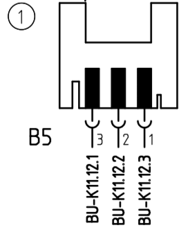
Sensor Salzmenge
