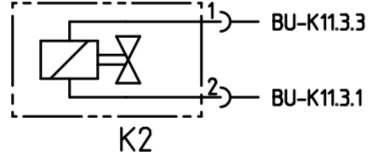
Auslassventil
