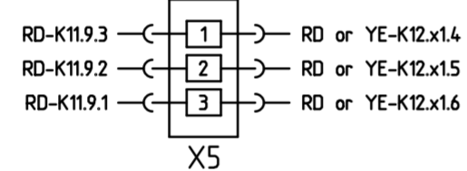
Kupplung
