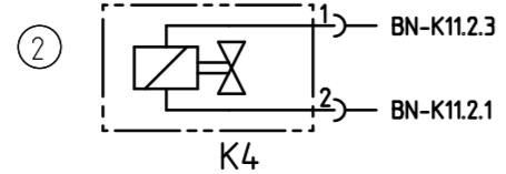
Fuellventil Warmwasser
