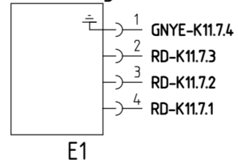
Temperatursensor
