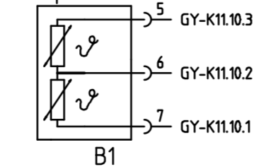
Temperatursensor
