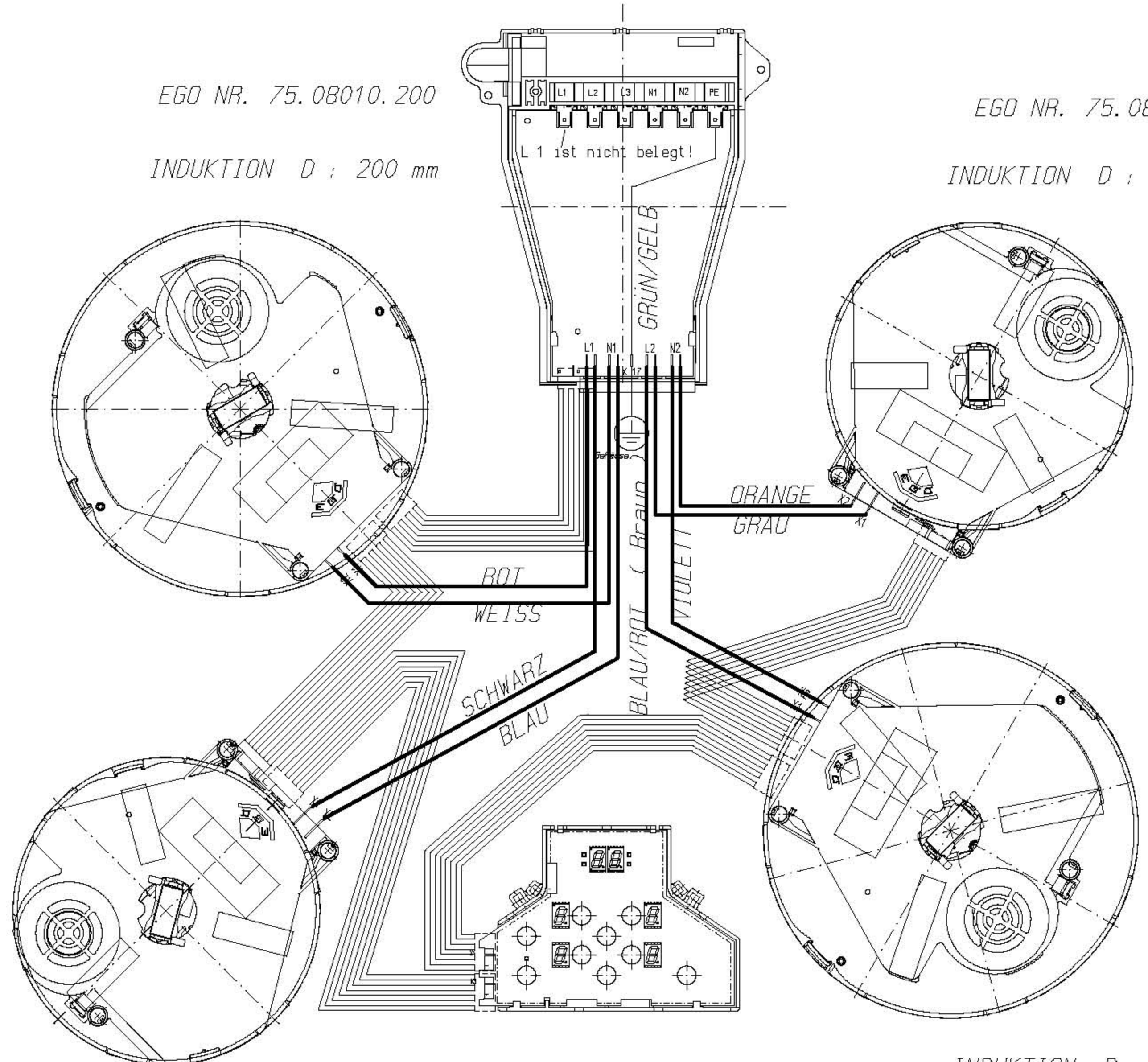
INDUKTION D : 200 mm EGO NR. 75.08010.200
