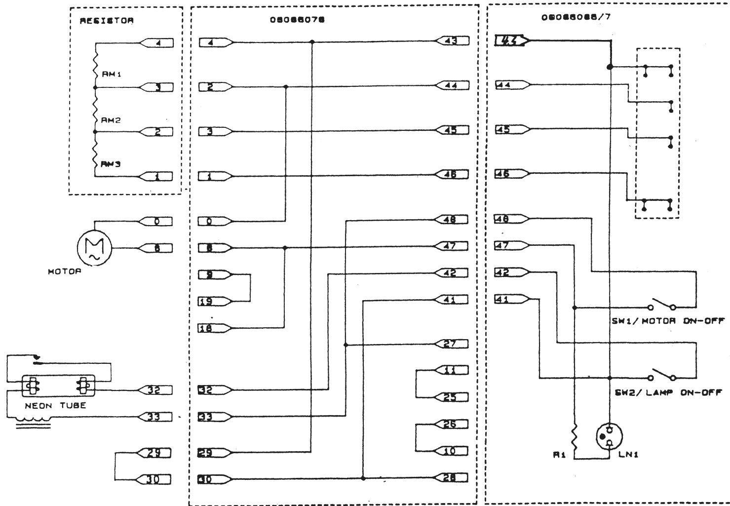
Schaltplan Nr. 00019
