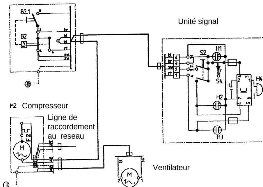
Schéma de connexions
