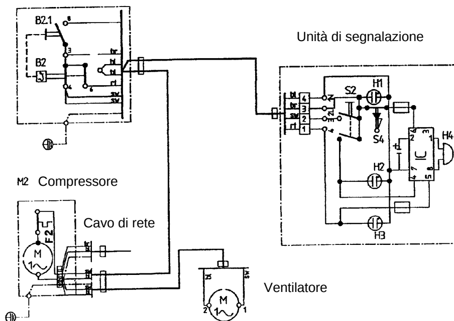
Schema degli allacciamento
