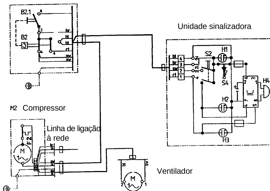
Esquema de ligação
