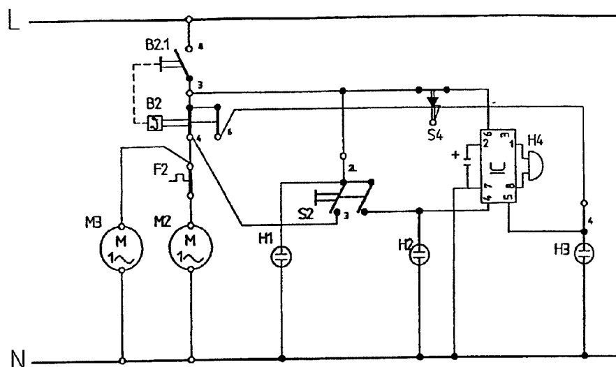
Esquema de circuito
