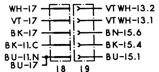
18 Steckgehaeuse + 19 Steckergehaeuse
