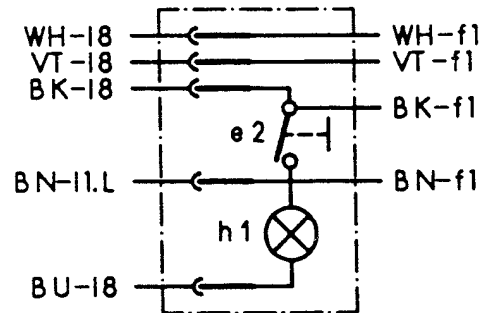
17 Steckbuchse
