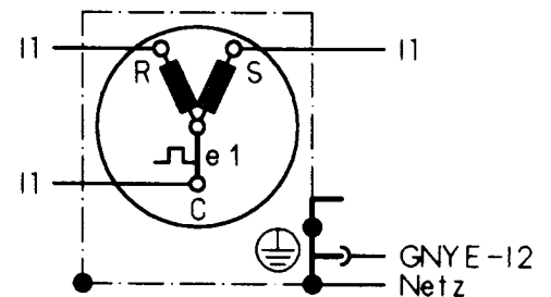
m1 Verdichter-Motor
