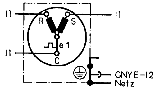
m1 Verdichter-Motor
