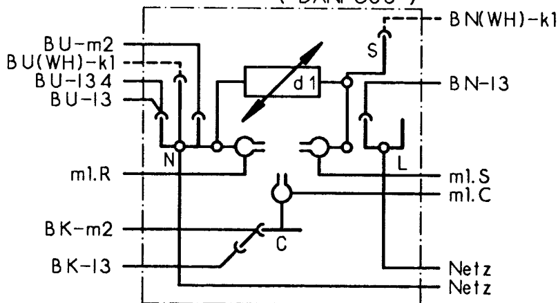
l1 Anschlussteil
