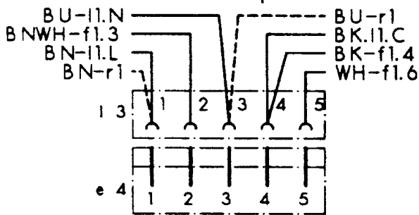
f1 Temperaturregler
