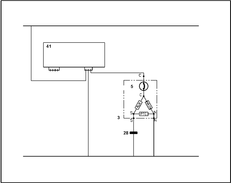
MORSETTIERA RAST5
