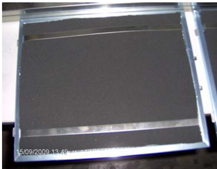
Abb. 2: Fettfilter mit Kohlefiltermatte und Befestigungsbügel
