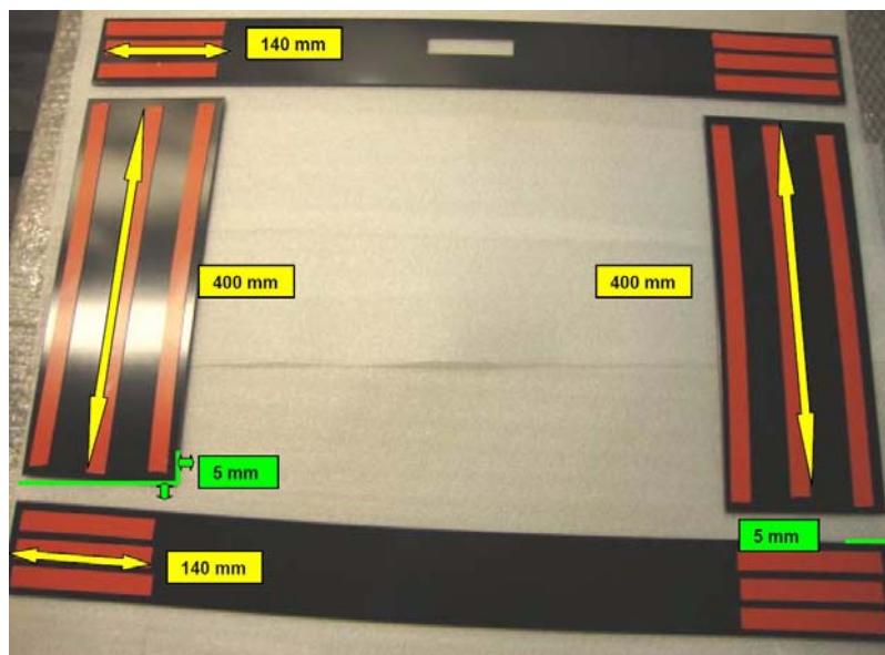
Abb. 1: Aufkleben des Klebebandes
