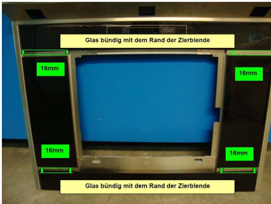
Abb. 2: Befestigung der Glasscheibe
