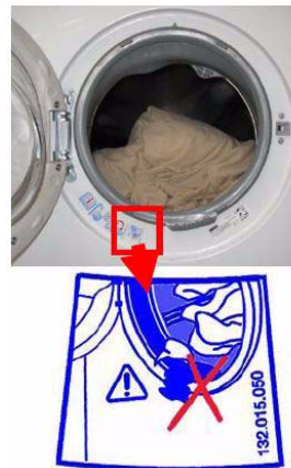
c) Hinweisaufkleber unterhalb der Türdichtung
