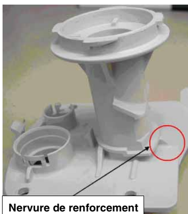
Couvercle modifié
