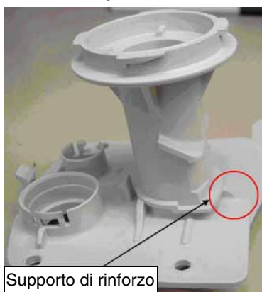
Nuovo coperchio
