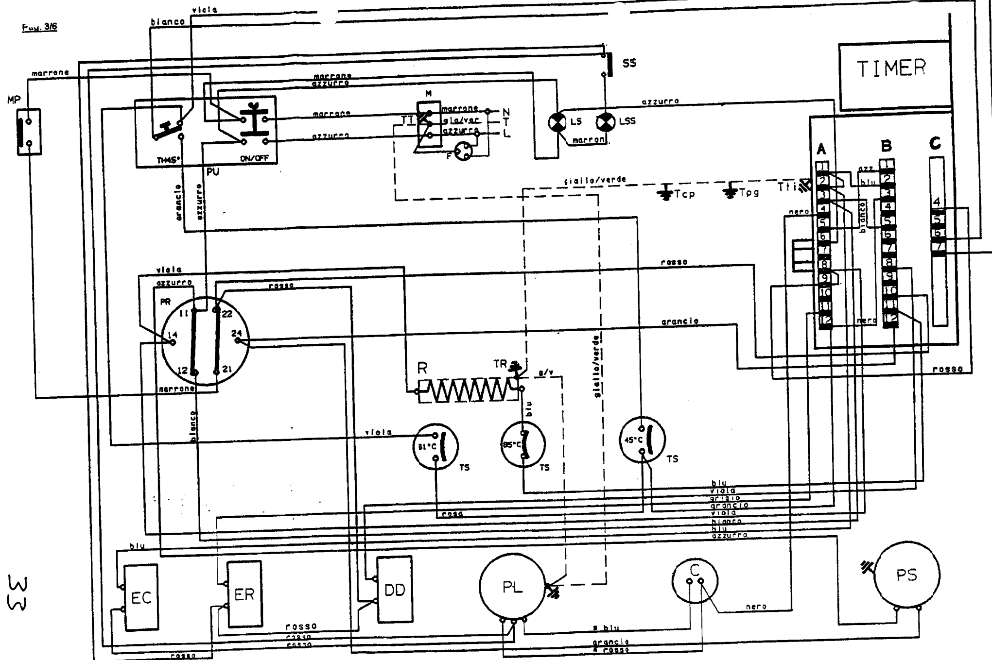
LAVAVAJILLAS / DISHWASHER MOD. TDW-45S DIAGRAMA DE CABLEADO / WIRING DIAGRAM
